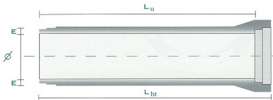
Coupe longitudinale d'un tuyau en béton de 2,42 m.
